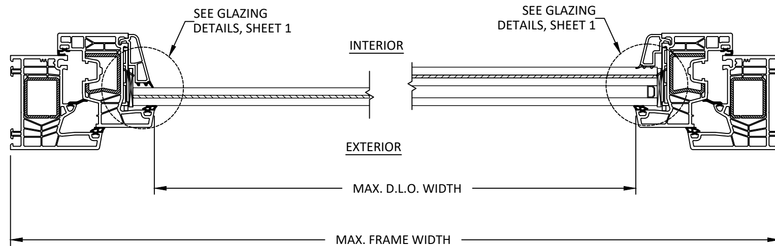
B 3 HORIZONTAL SECTION BALCONY DOOR
